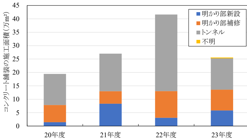
直轄国道におけるコンクリート舗装の施工面積の推移
