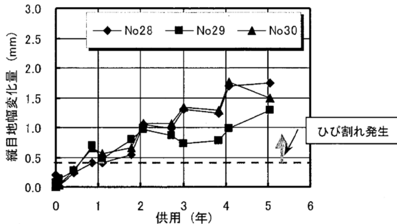
図6-3 縦方向目地の目地幅変化量の経時変化
