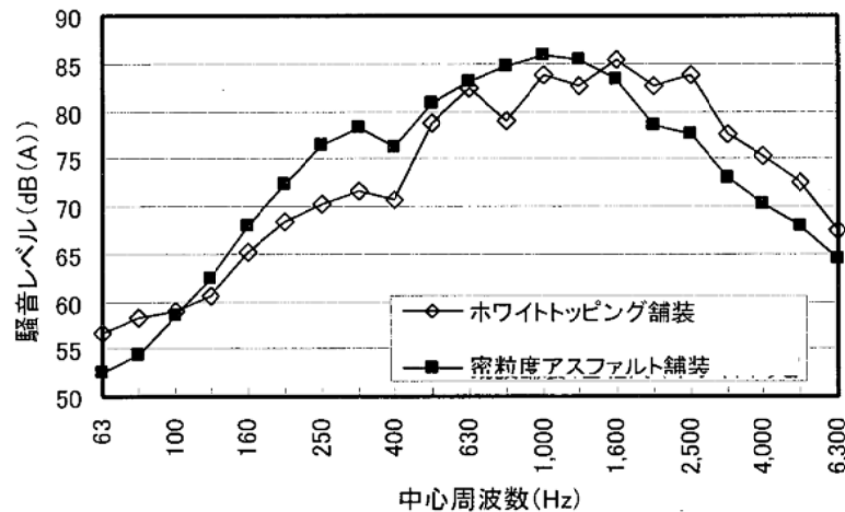
図6-10 1/3オクターブバンド分析による騒音レベルの一例（供用後4年時測定）
