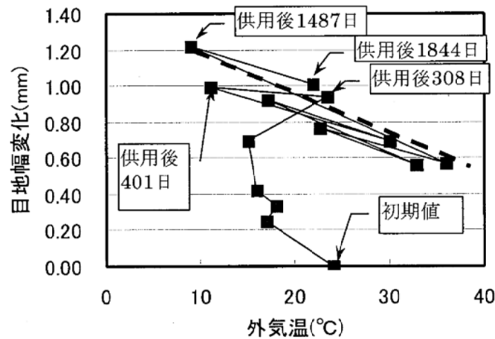
図6-4 目地幅変化量と外気温度の関係
