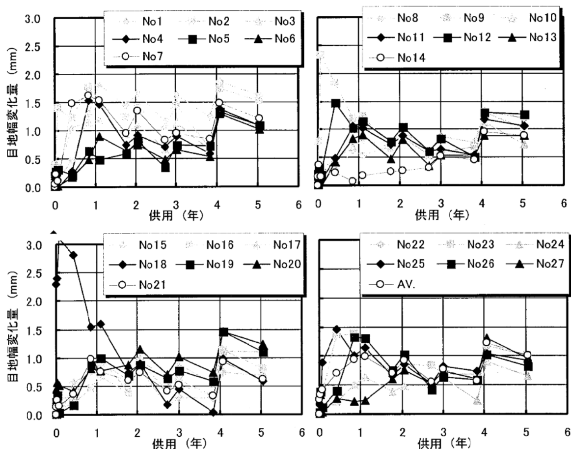
図 6-2 横方向目地の目地幅変化量の経時変化
