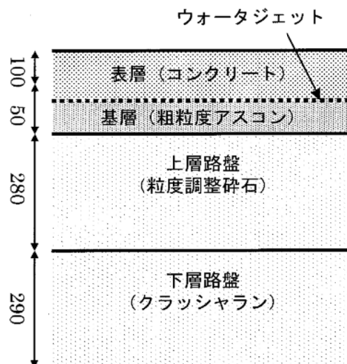
図 3-4 本試験舗装の設計断面 (mm)
