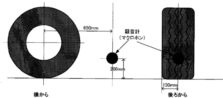
図 5-8 マイクロフォン設置位置
