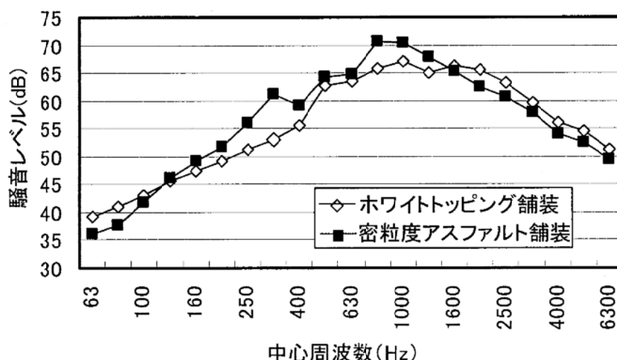
図6-12 1/3オクターブバンド分析の一例（騒音ピークレベル、供用後4年時測定）
