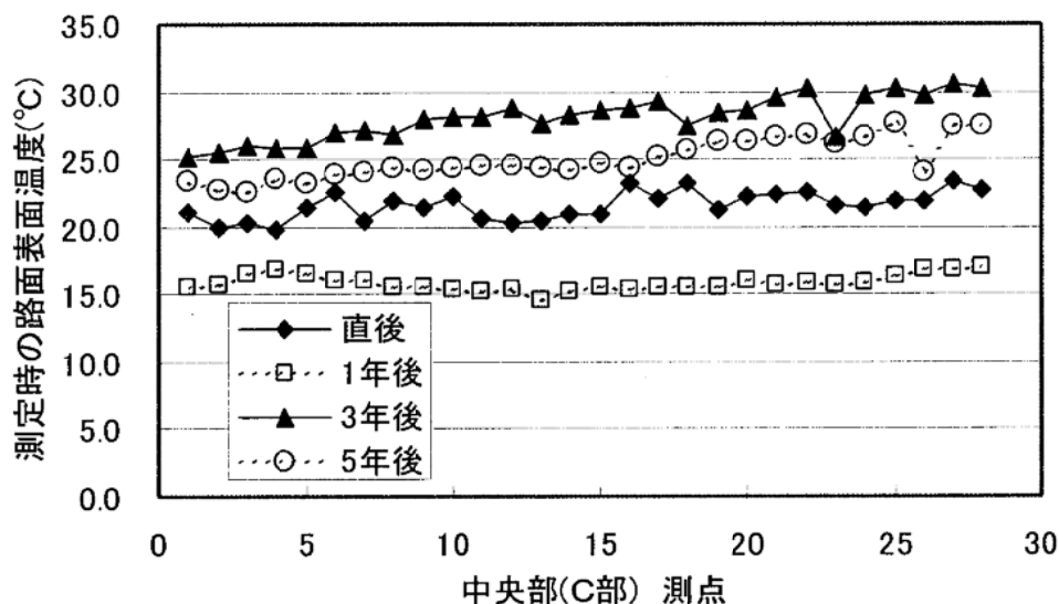
図 6-6 路面温度の測定結果
