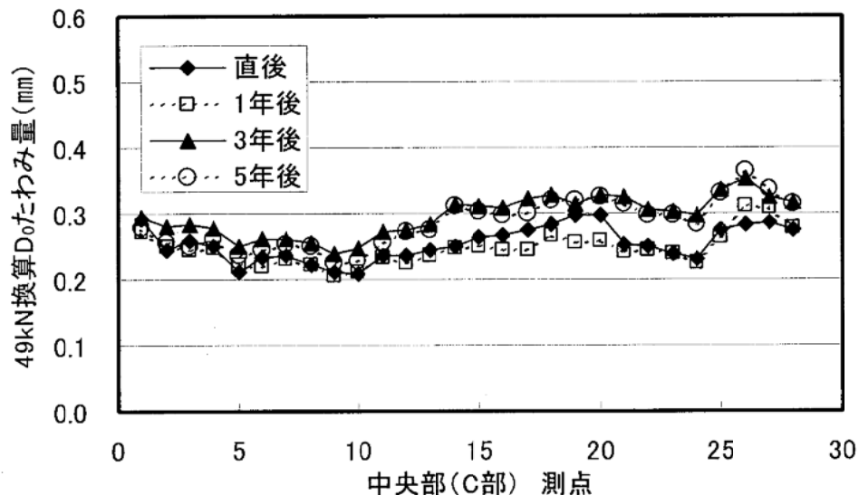
図 6-5 版中央部の载荷版直下 D_0 たわみ量の測定結果
